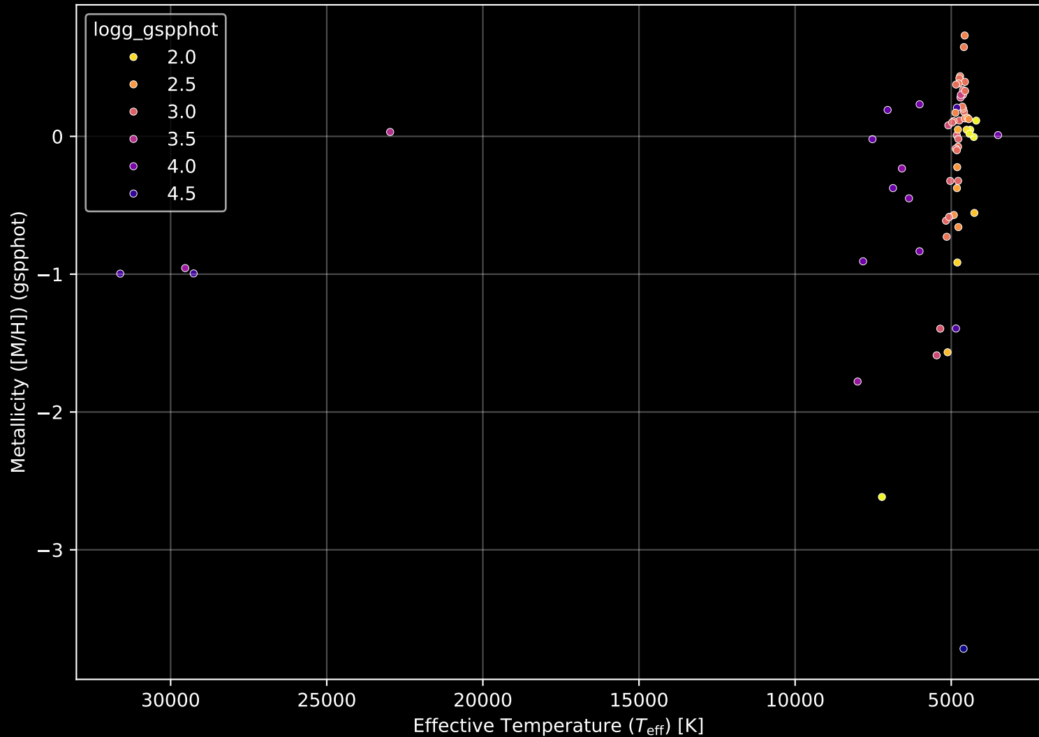
APOGEE DR17 Field: [LMC9] Stellar Population Parameters (n= 67)
